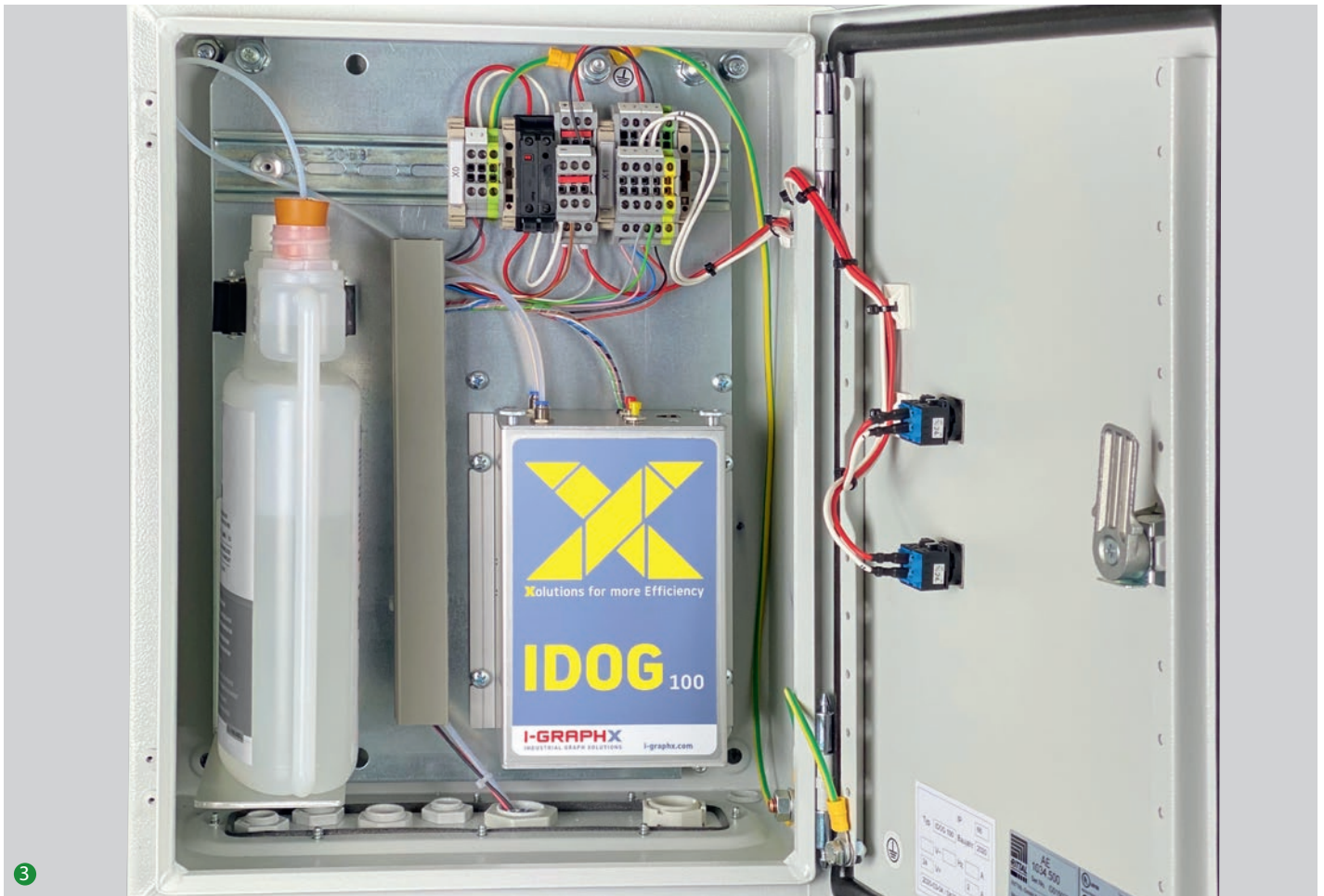
3 Schaltschrank mit Vorratsflasche und Controller Box I-DOG 100
